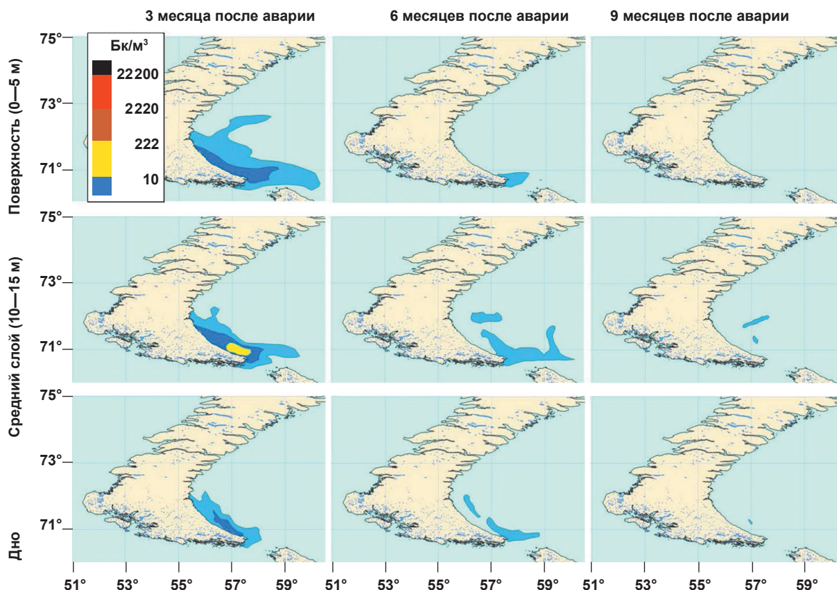
Рис. 5. Среднесрочный прогноз распространения загрязнения при максимальном залповом выбросе 6 Тбк 137 Cs из находящейся на дне АПЛ К-27. Расчеты авторов Fig. 5. Medium-term forecast of contamination propagation in result of UCR with release 6 Tb 137 Cs, at K-27 at the bottom. Authors calculations
