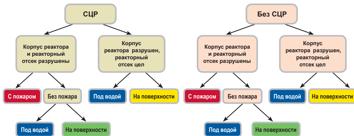
Рис. 3. Варианты гипотетических аварий ЗЯРОО. Составлено авторами Fig. 3. Options of hypothetical DNRHO accidents. Compiled by the authors
