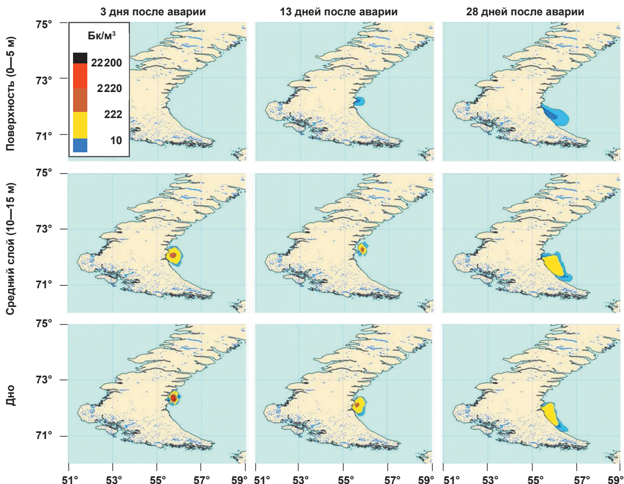
Рис. 4. Распространение загрязнения в результате СЦР с выбросом 6 Тб на АПЛ К-27 при нахождении ее на дне. Расчет авторов
